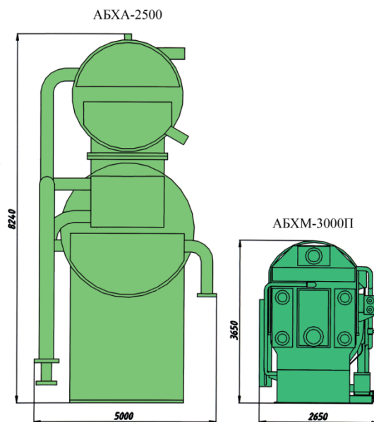
Рис. 3. Сравнительные размеры АБХМ российского производства разных лет (слева – выпускаемые с 1964 по 1991 гг., справа – с 2000 г. по н.в.).
