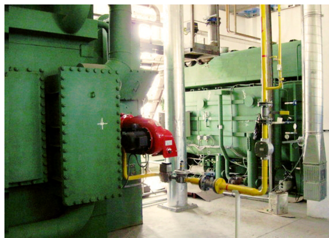
Холодильная станция на базе двух машин с огневым обогревом (природный газ) АБХМ-1500Тс мощностью 3000 кВт для линии розлива минеральной воды в ООО "Карачинский источник"
