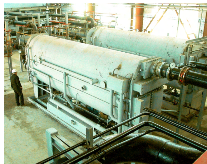
Холодильная станция на базе двух машин с паровым обогревом АБХМ-1500П мощностью 3500 кВт для линии производства хрома в ОАО "Полема", г. Тула.
